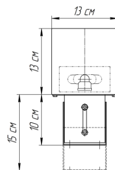
Исполнение "рв" (регулируемая высота)
