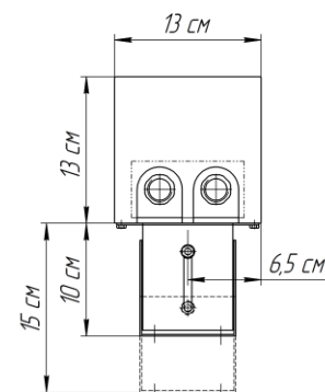
Исполнение "рв" (регулируемая высота)
