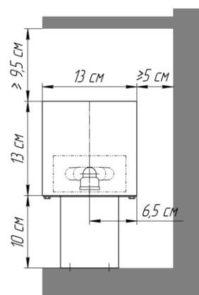
Исполнение "нв" (нерегулируемая высота)
