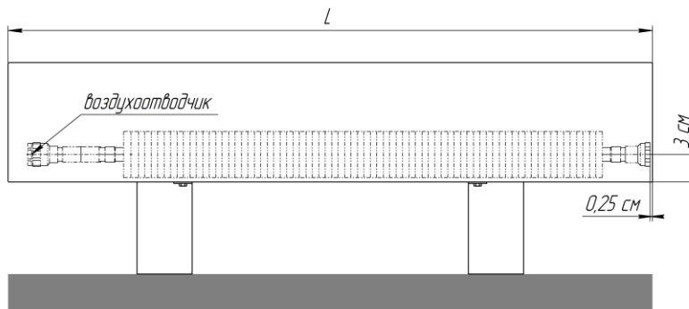
Вид для исполнения "нв" (нерегулируемая высота)
